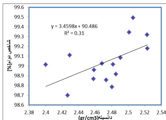
شکل ۳- رابطه بین دانسیته و شاخص دوام (سازند آبدراز)
