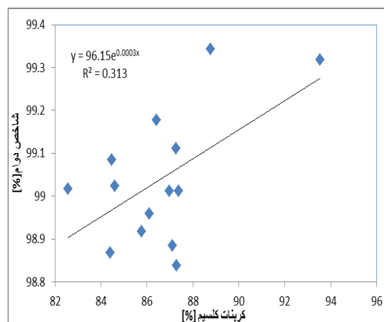
شکل ۷- رابطه بین کربنات کلسیم و شاخص دوام (سازند آبدراز)
