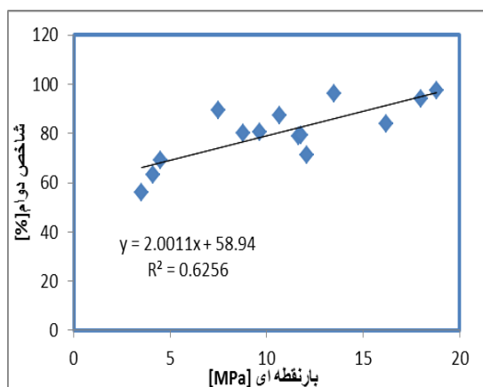
شکل ۶- رابطه بین شاخص بار نقطه ای و شاخص دوام (سازند آب تلخ)
