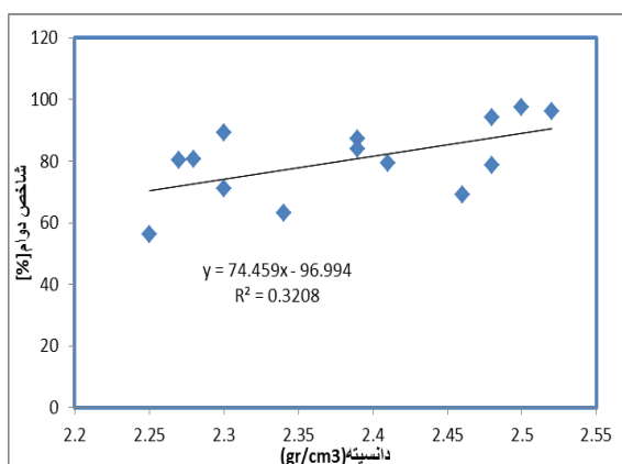
شکل ۴- رابطه بین دانسیته و شاخص دوام (سازند آب تلخ)
