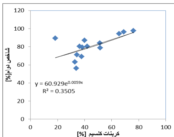
شکل ۸- رابطه بین کربنات کلسیم و شاخص دوام (سازند آب تلخ)
