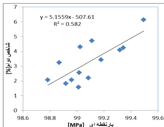
شکل ۵- رابطه بین شاخص بار نقطه ای و شاخص دوام (سازند آبدراز)
