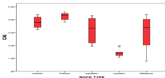
شکل ۵- نمودار جعبه‌ای داده های آزمون سرشار (CAI) بر روی سنگ‌های مختلف
