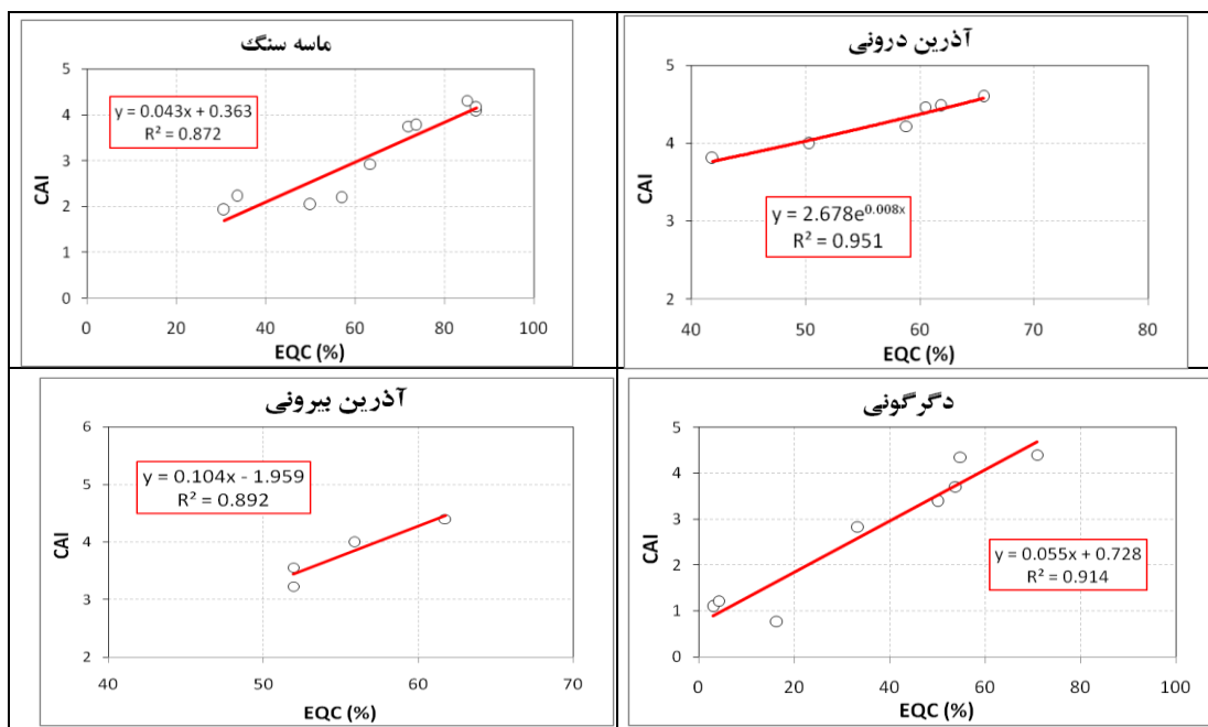
شکل ۶- نمودار پراکنش و رگرسیون بین CAI و EQC برای هر یک از انواع سنگ‌های مختلف
