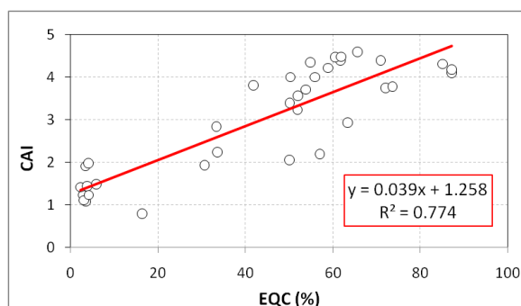
شکل ۷- نمودار پراکنش و رگرسیون بین CAI و EQC برای همه انواع سنگ‌های مختلف
