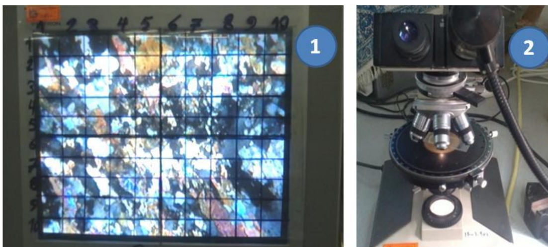
شکل ۳- آزمون پتروگرافی در مقطع نازک: (۱- میکروسکوپ مجهز به دوربین، ۱- تجزیه و تحلیل پتروگرافی به وسیله میکروسکوپ و مانیتور)
