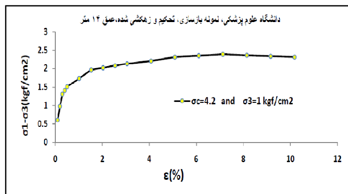
شکل ۸ منحنی تغییرات تنش - کرنش محوری نمونه بازسازی و زهکشی شده، دانشگاه علوم پزشکی کرمان عمق ۱۰.۴۵-۱۰ متر
