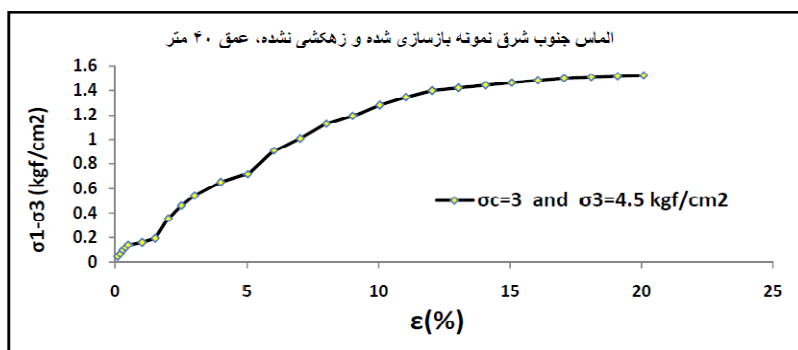
شکل ۲ منحنی های تنش - کرنش محوری نمونه بازسازی شده و زهکشی نشده، سایت الماس جنوب شرق عمق ۴۰ متر
