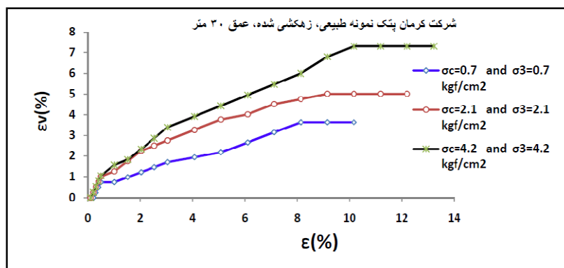
شکل ۱۲ منحنی های کرنش محوری - کرنش حجمی نمونه های طبیعی زهکشی شده، شرکت کرمان پتک عمق ۳۰-۳۰.۴۵ متر
