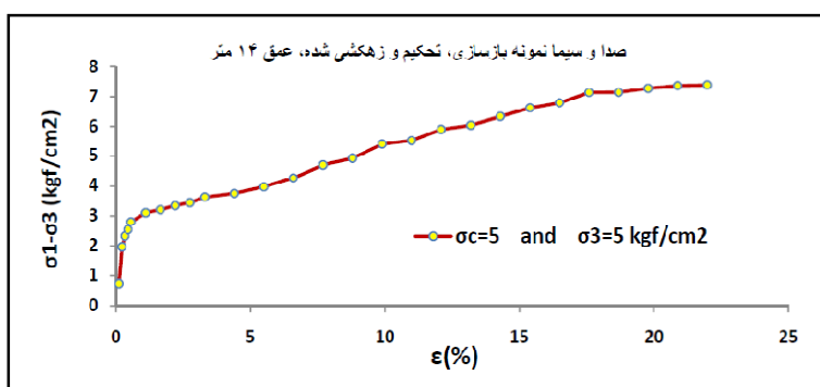
شکل ۹ منحنی تغییرات تنش - کرنش محوری نمونه بازسازی و زهکشی شده، سایت سازمان صدا و سیما عمق ۱۴.۴۵-۱۴ متر
