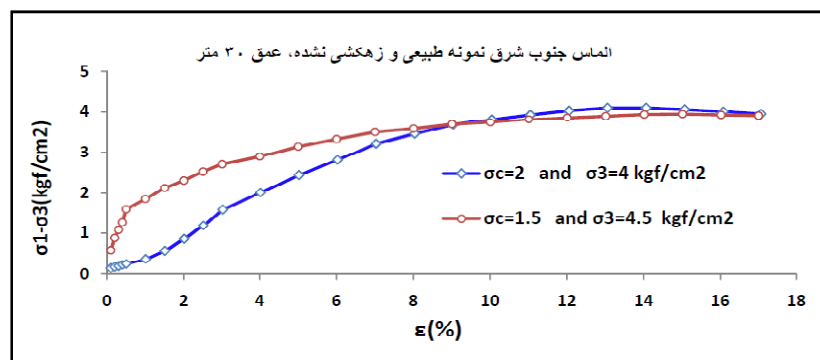
شکل ۳ منحنی تغییرات تنش - کرنش محوری نمونه های طبیعی و زهکشی نشده، سایت الماس جنوب شرق عمق ۳۰ متر
