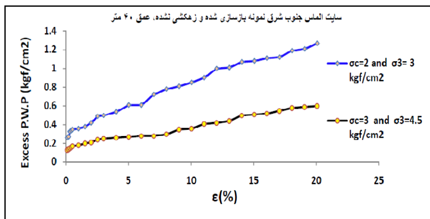
شکل ۱۰ منحنی های کرنش محوری - فشار منفذی نمونه های بازسازی شده زهکشی نشده، الماس جنوب شرق عمق ۴۰ متر
