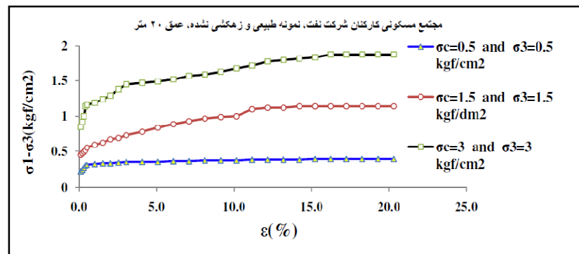
شکل ۴ منحنی های تنش - کرنش نمونه های طبیعی زهکشی نشده، مجتمع مسکونی کارکنان شرکت نفت عمق ۲۰-۲۰.۴۵ متر
