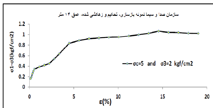
شکل ۷ منحنی تغییرات تنش - کرنش محوری نمونه بازسازی و زهکشی شده، سایت سازمان صدا و سیما عمق ۱۴-۱۴.۴۵ متر
