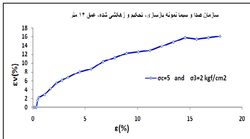
شکل ۱۱ منحنی کرنش محوری - کرنش حجمی نمونه بازسازی و زهکشی شده، سایت سازمان صدا و سیما عمق ۱۴-۱۴.۴۵ متر
