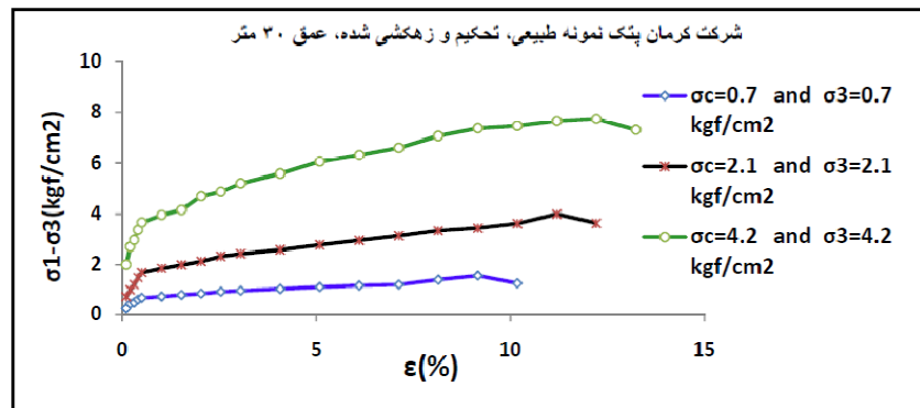
شکل ۱۰ منحنی تغییرات تنش - کرنش محوری نمونه های طبیعی زهکشی شده، سایت شرکت کرمان پتک عمق ۳۰-۳۰.۴۵ متر
