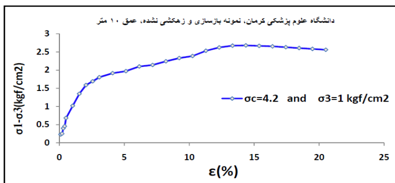
شکل ۱ منحنی تنش - کرنش محوری نمونه بازسازی شده و زهکشی نشده، سایت دانشگاه علوم پزشکی کرمان عمق ۱۰ متر
