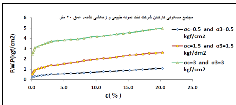
شکل ۱۲ منحنی های کرنش - فشار منقذی نمونه های طبیعی زهکشی نشده، مجتمع کارکنان شرکت نفت عمق ۲۰-۲۰.۴۵ متر
